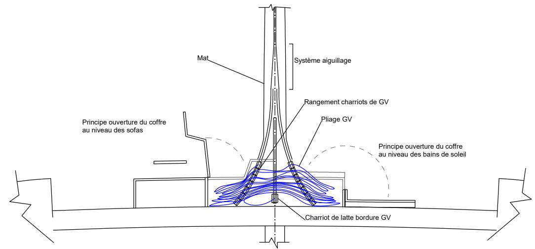
Principe affalage et rangement GV dans coffres sofas
